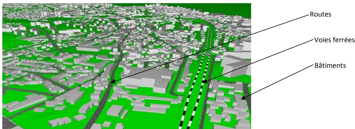
Figure 13 : Représentation 3D du modèle de calcul acoustique
